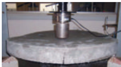
Ensayo RDP de absorción de energía.
