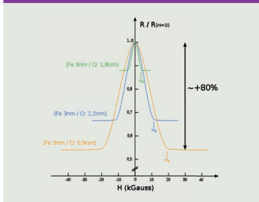
Figura 1. a) Nanoestructura con comportamiento Magneto-resistivo Gigante: característica de la magneto-resistencia versus intensidad de Campo Magnético
